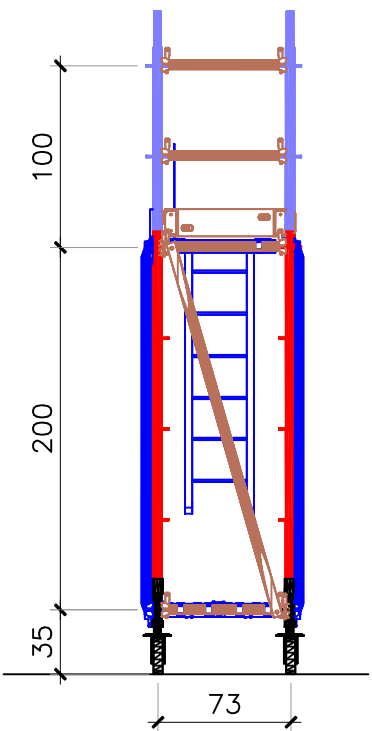
SECCION A
