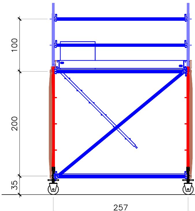
SECCION B
