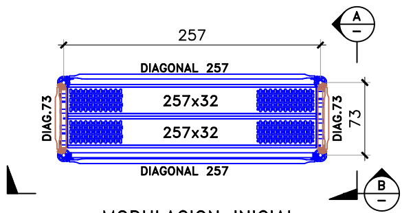
MODULACION INICIAL
