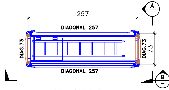
MODULACION FINAL
